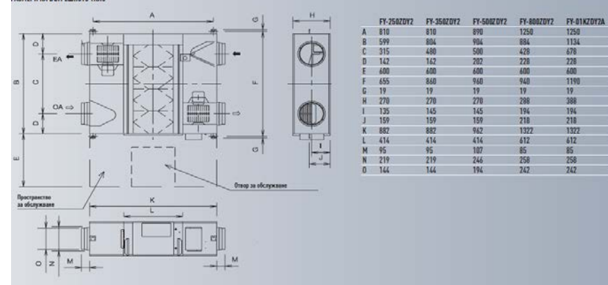
РАЗМЕРИ НА ВЪТРЕШНОТО ТЯЛО
