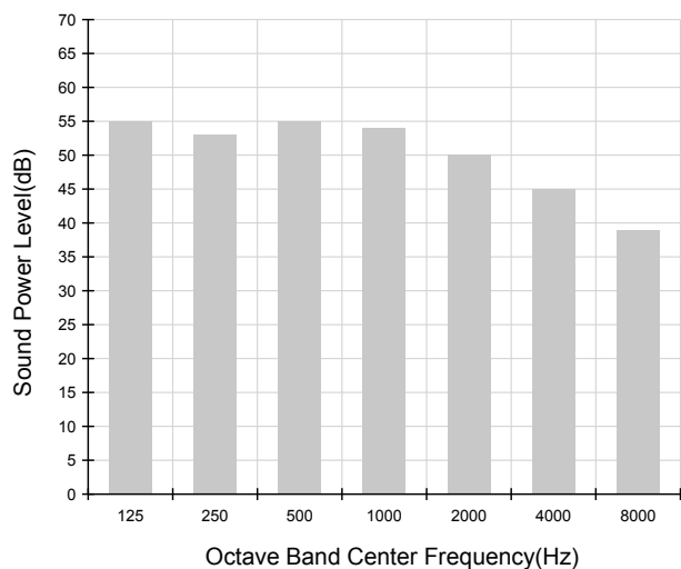
3) AC100HBMDKH/EU (ODU : AC100HCADNH/EU)
