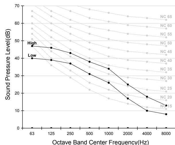
4) AC140HBMDKH/EU (ODU : AC140HCADKH/EU)
