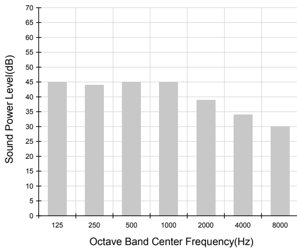
1) AC052HBMDKH/EU (ODU : AC052HCADKH/EU)
